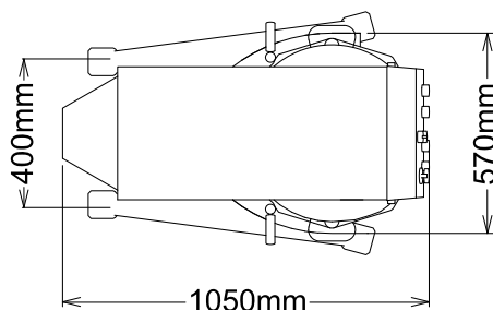
Boven aanzicht
